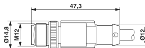
Stecker gerade M12 / IP67 Anzugsdrehmoment 0,4 Nm
