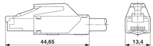
Stecker gerade RJ45 / IP20
