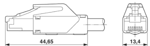
Stecker gerade RJ45 / IP20
