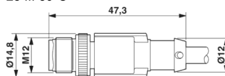
Stecker gerade M12 / IP67 Anzugsdrehmoment 0,4 Nm
