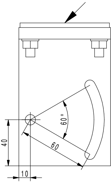
Montagesite für das Metis Kühlgehäuse
